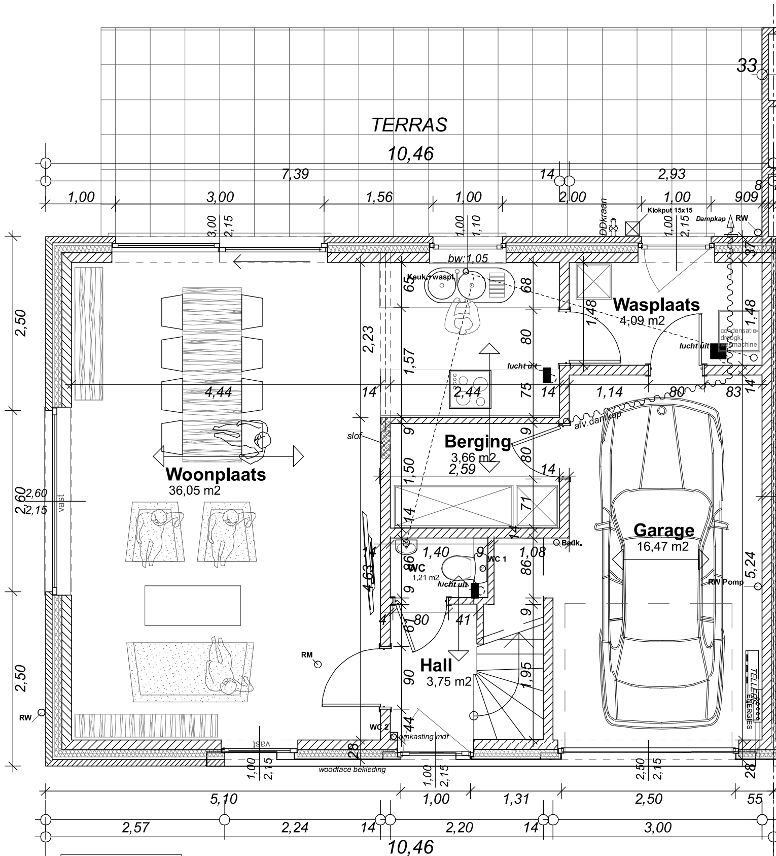
WONING 3
